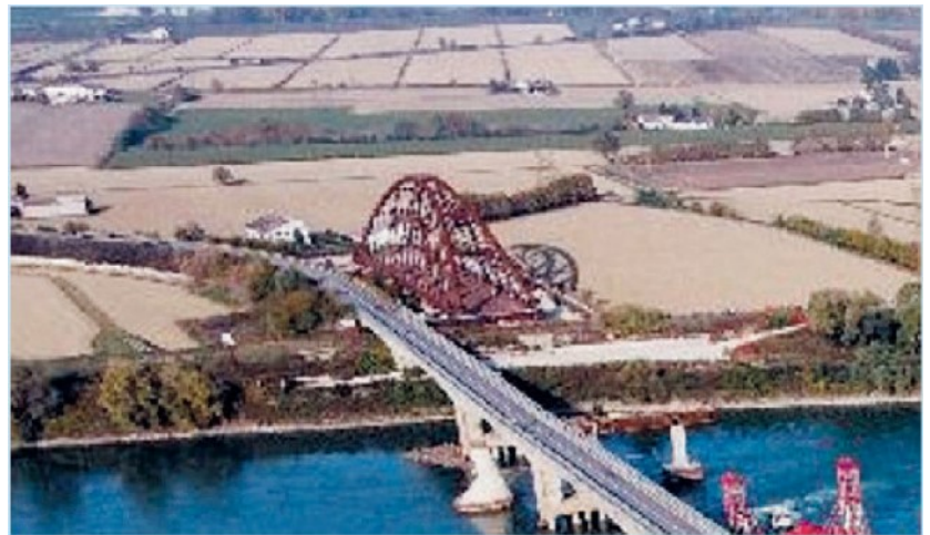
L'arcata del lato bagnolese che sarà varata nelle prossime settimane (foto Matteo Sessa)
